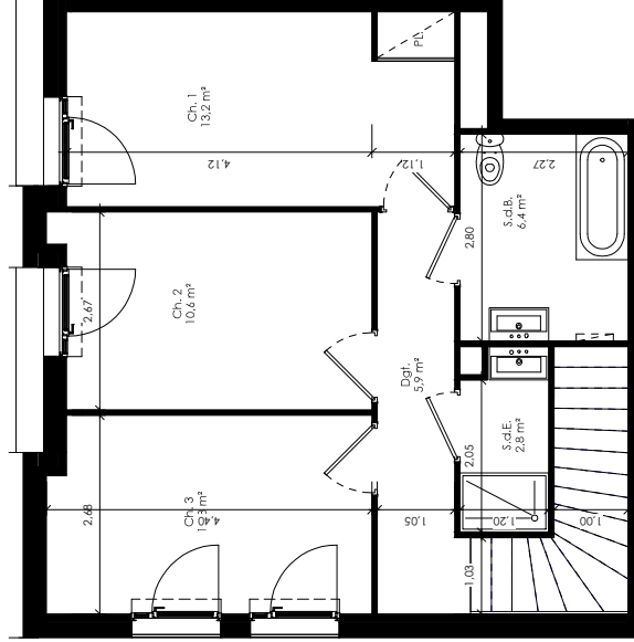
DUPLEX - NIVEAU HAUT
