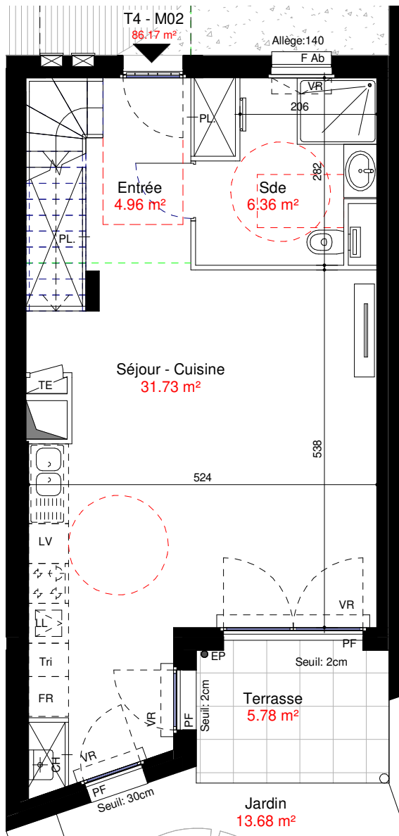
PLAN DU REZ-DE-CHAUSSEE
