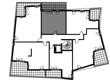
Plan de niveaux
